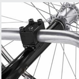
Tube d'essieu oversize réglable pour un réglage optimal du centre de gravité
